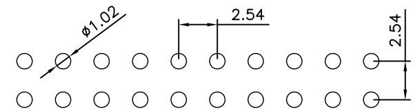
P.C.B LAYOUT
