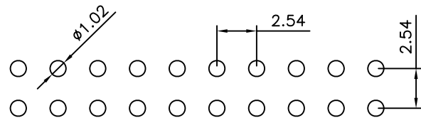
P.C.B LAYOUT
