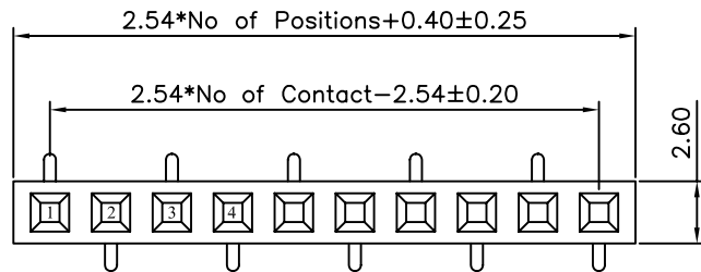
SMT B Type
