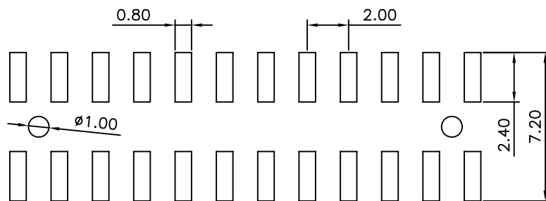
P.C.B LAYOUT
