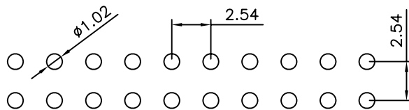
P.C.B LAYOUT
