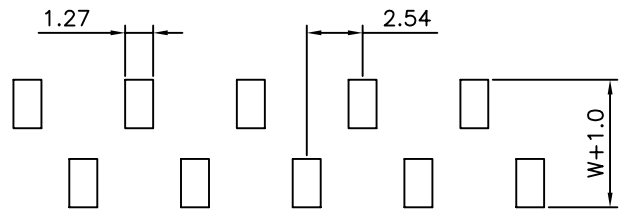
P.C.B LAYOUT
