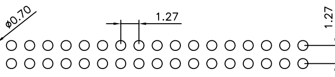
P.C.B LAYOUT
