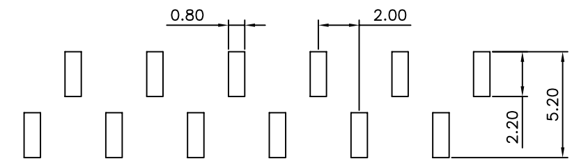
P.C.B LAYOUT
