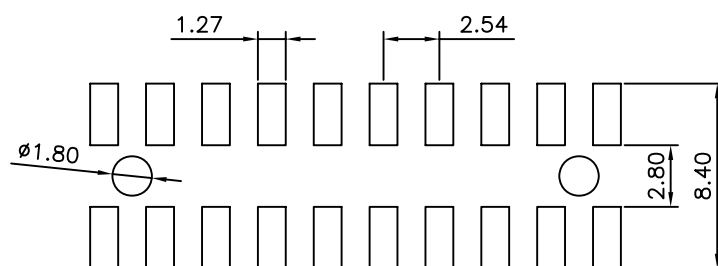
P.C.B LAYOUT
