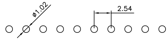
P.C.B LAYOUT
