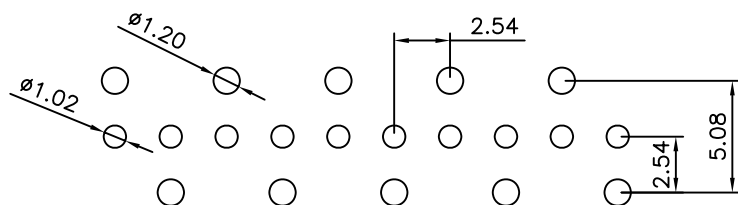
P.C.B LAYOUT
