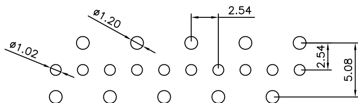
P.C.B LAYOUT
