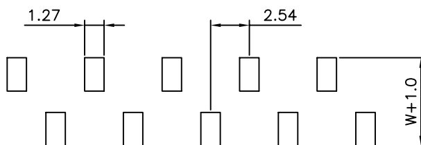
P.C.B LAYOUT
